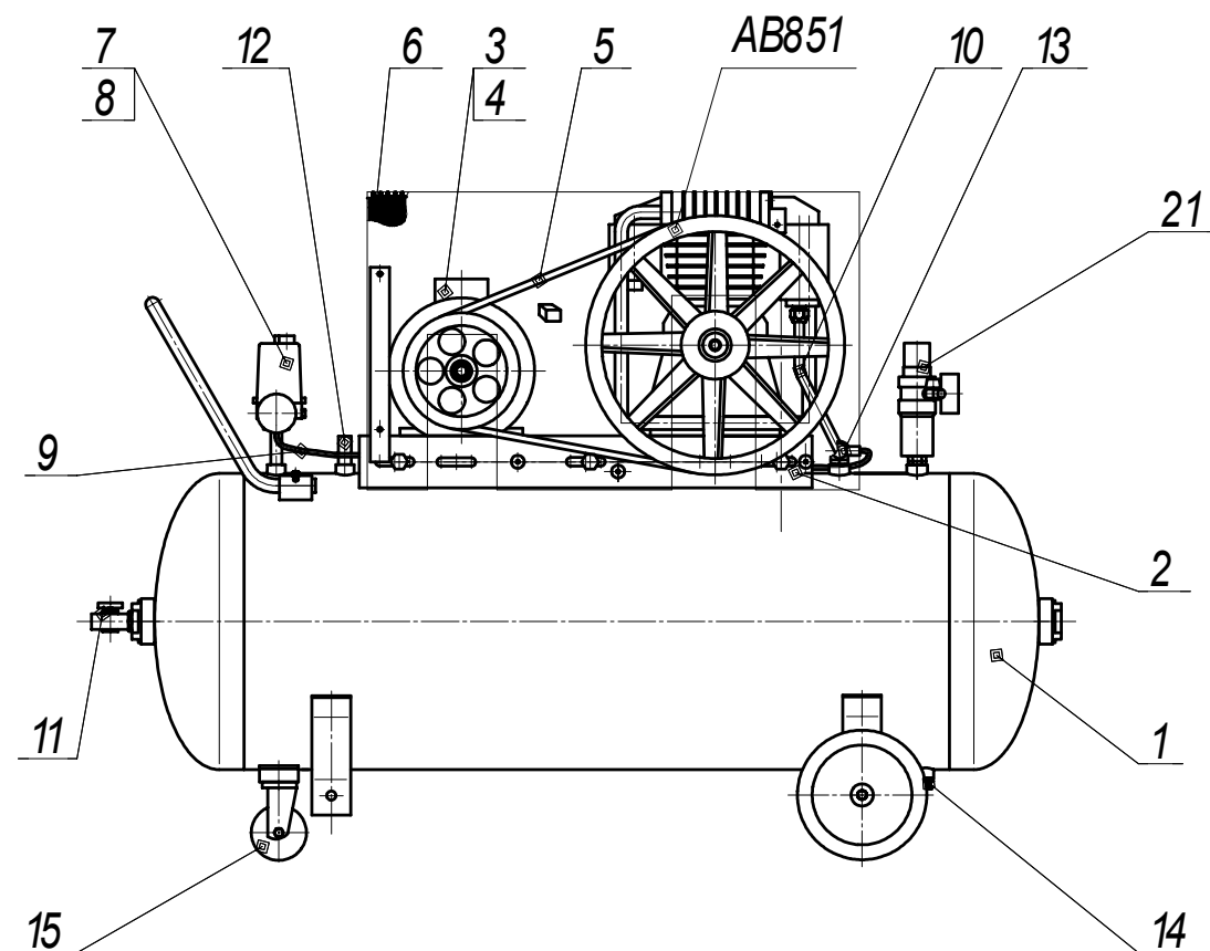
Рисунок 2 – Общий вид компрессора СБ4/С-270.АВ850, СБ4/Ф-270.АВ850, СБ4/Ф-270.АВ850/15, СБ4/Ф-270.АВ850/16
