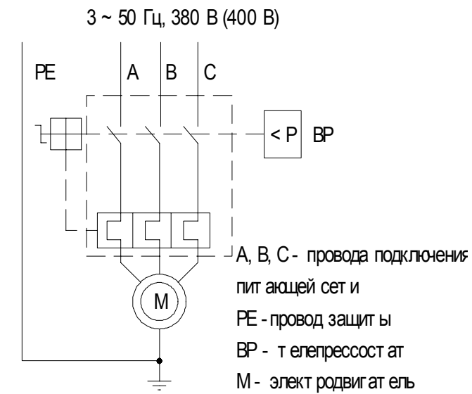
Рисунок 7 – Схема электрическая принципиальная для СБ4/С-100.АВ850, СБ4/С-270.АВ850, СБ4/Ф-270.АВ850, СБ4/Ф-270.АВ850В, СБ4/Ф-270.АВ850/15, СБ4/Ф-270.АВ850/16, СБ4/Ф-500.АВ850, СБ4/Ф-500.АВ850/15, СБ4/Ф-500.АВ850/16
