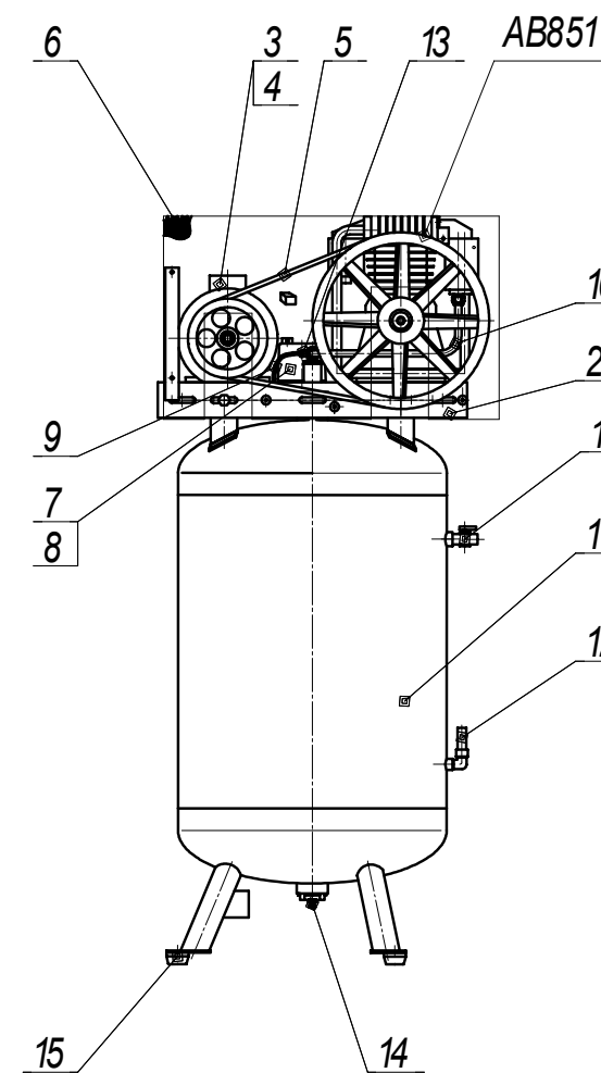
Рисунок 4 – Общий вид компрессора СБ4/Ф-270.АВ850В
