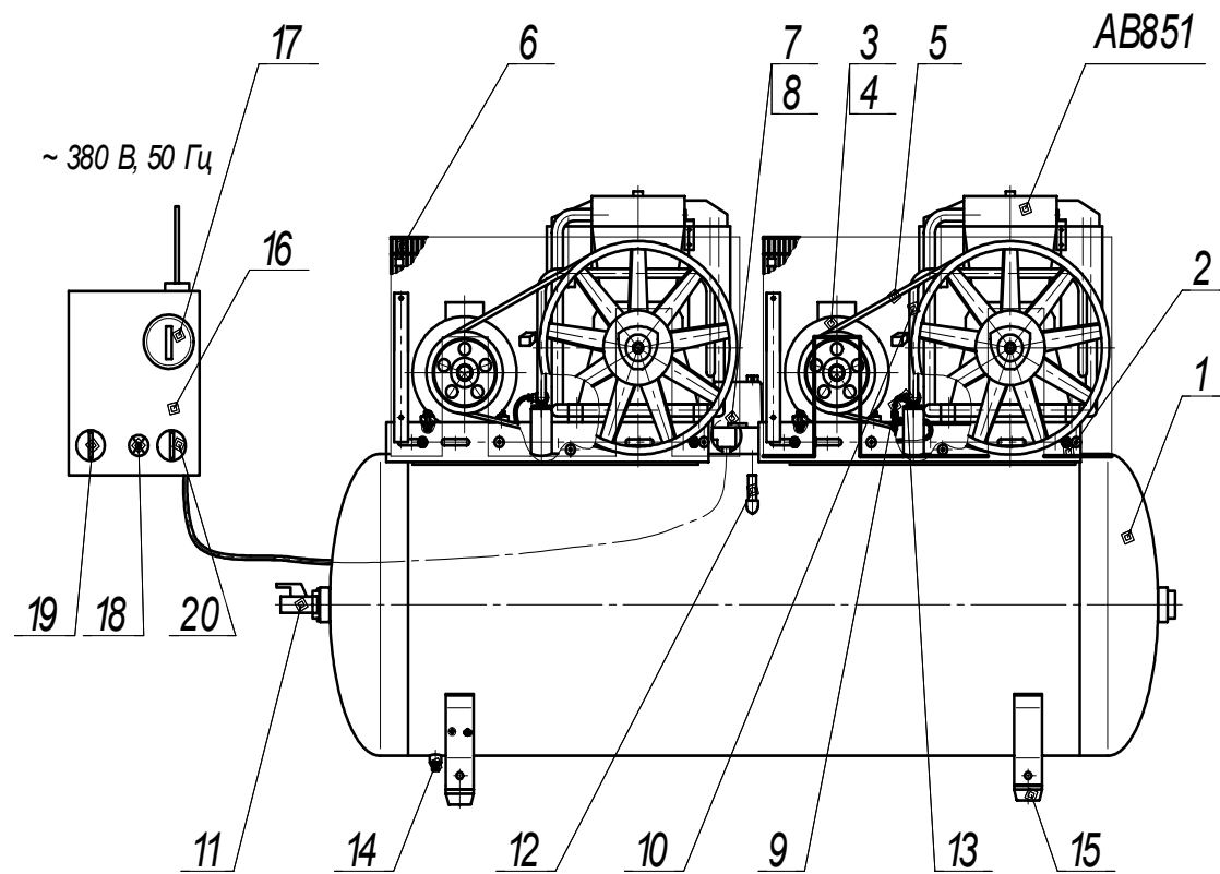
Рисунок 5 – Общий вид компрессора СБ4/Ф-500.АВ850Т, СБ4/Ф-500.АВ850Т/15, СБ4/Ф-500.АВ850Т/16
