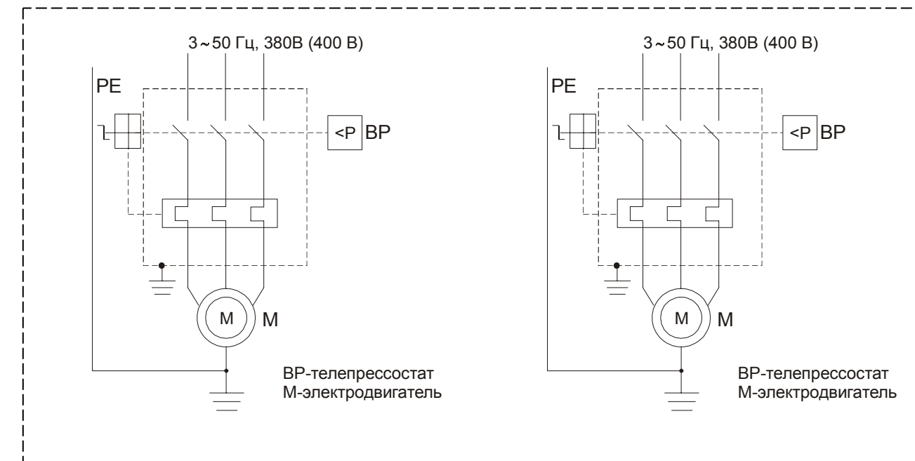
Рисунок 8 – Схема электрическая принципиальная для СБ4/Ф-500.АВ850ТБ
