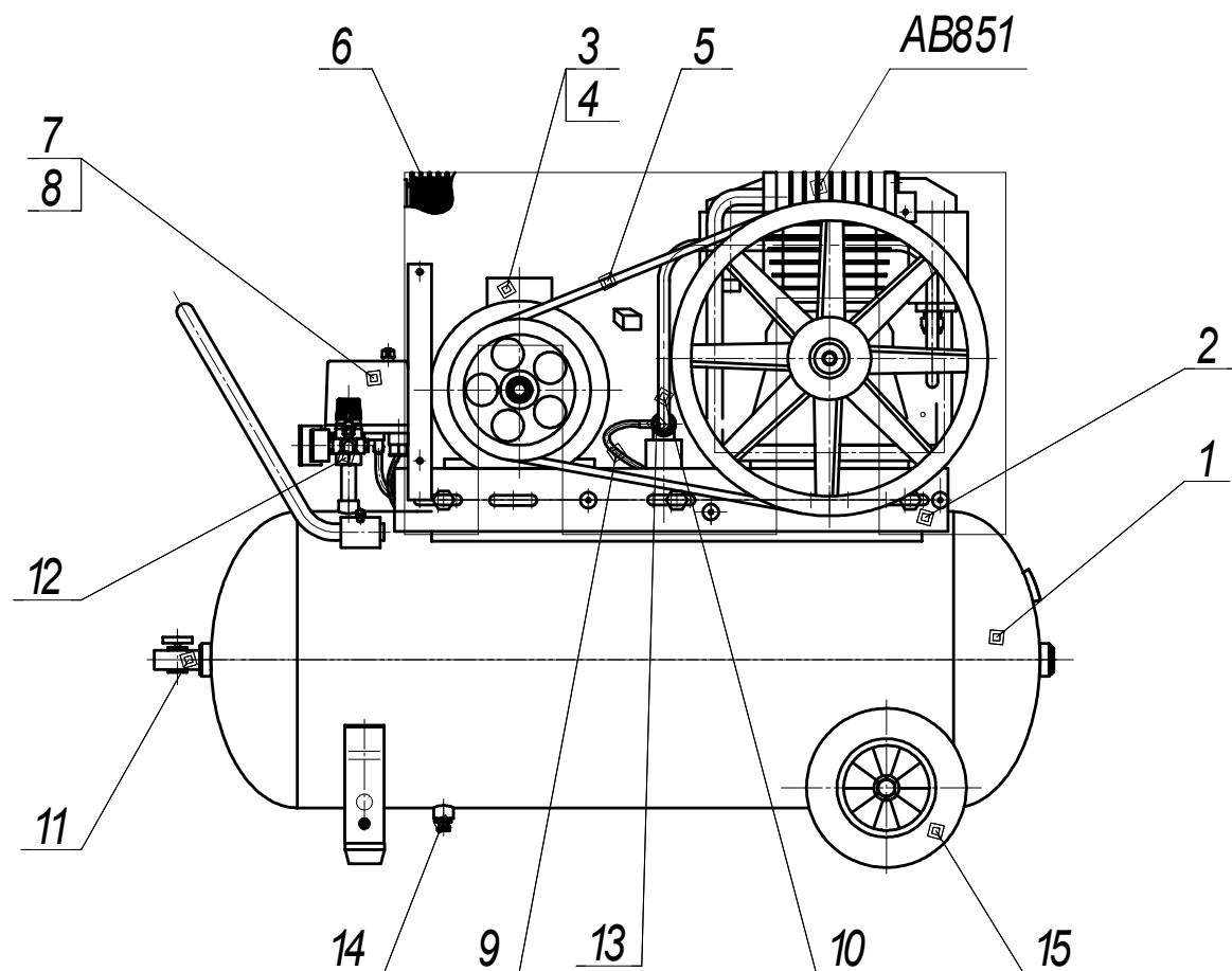
Рисунок 1 – Общий вид компрессора СБ4/С-100. АВ850
