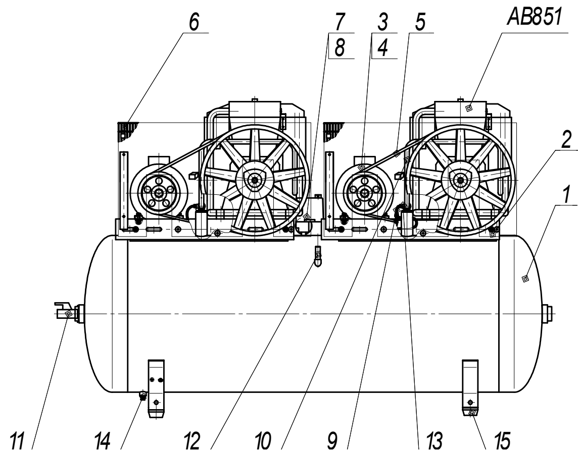
Рисунок 6 – Общий вид компрессора СБ4/Ф-500.АВ850ТБ
